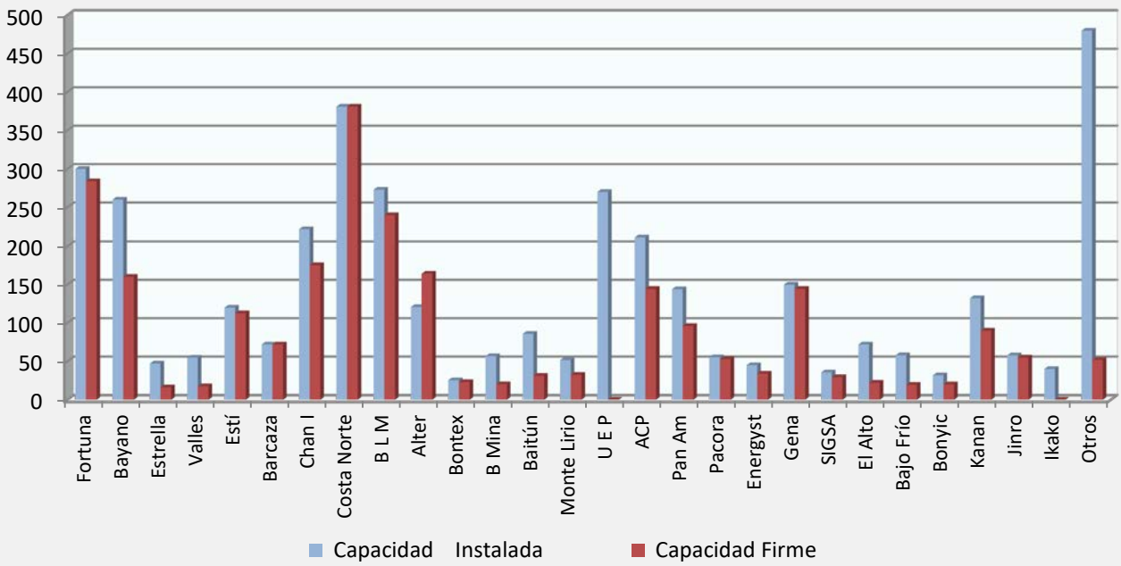
CAPACIDAD INSTALADA Y CAPACIDAD FIRME POR PLANTA (MW) 2021
