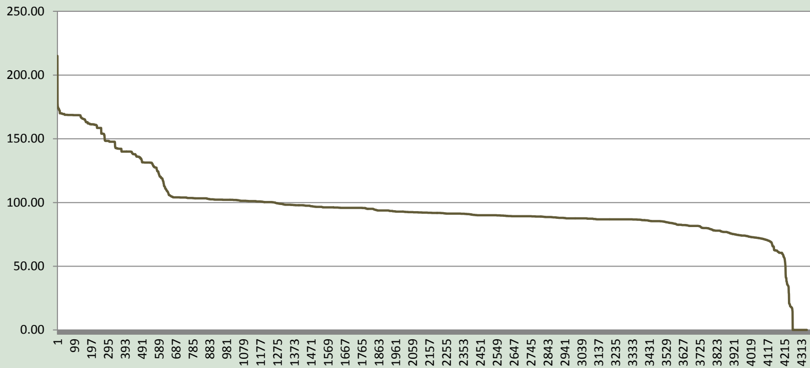
GRÁFICO No. 45 DURACIÓN DEL PRECIO HORARIO EN EL MERCADO OCASIONAL Enero - Junio 2015 (B/. / MWh)
