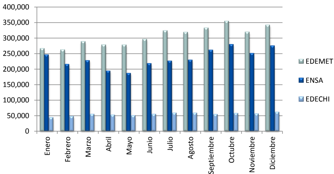
GRÁFICO No. 39 ENERGÍA ADQUIRIDA EN CONTRATOS 2014
