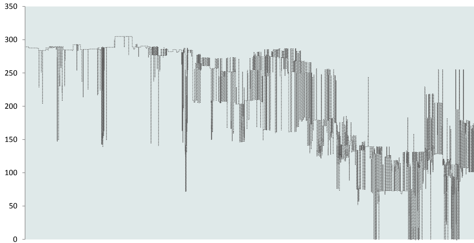
GRÁFICO No. 43 PRECIO HORARIO DE LA ENERGÍA EN EL MERCADO OCASIONAL Año 2014 (B/. / MWh)
