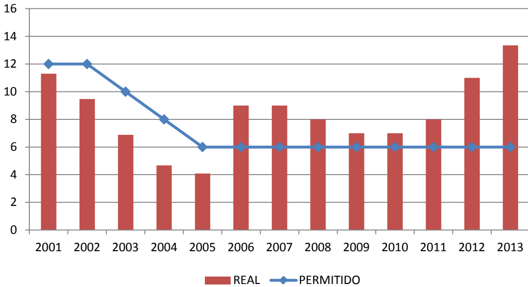
GRÁFICO No. 46 SAIFI DE ENSA EN CENTROS URBANOS AÑOS 2001 - 2013
