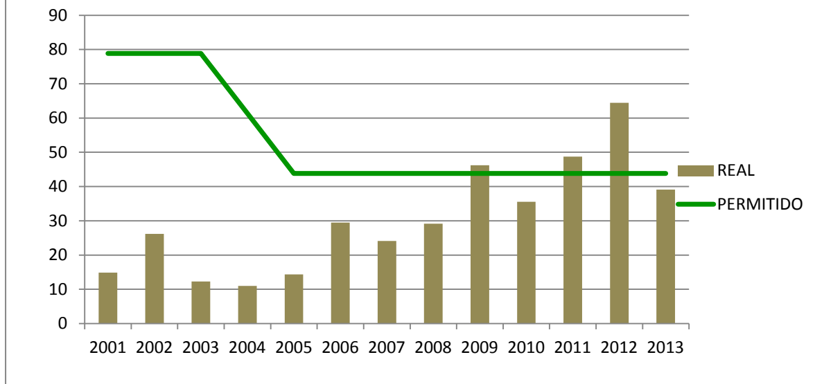
GRÁFICO No. 57 SAIDI DE EDECHI EN CENTROS RURALES AÑOS 2001 - 2013
