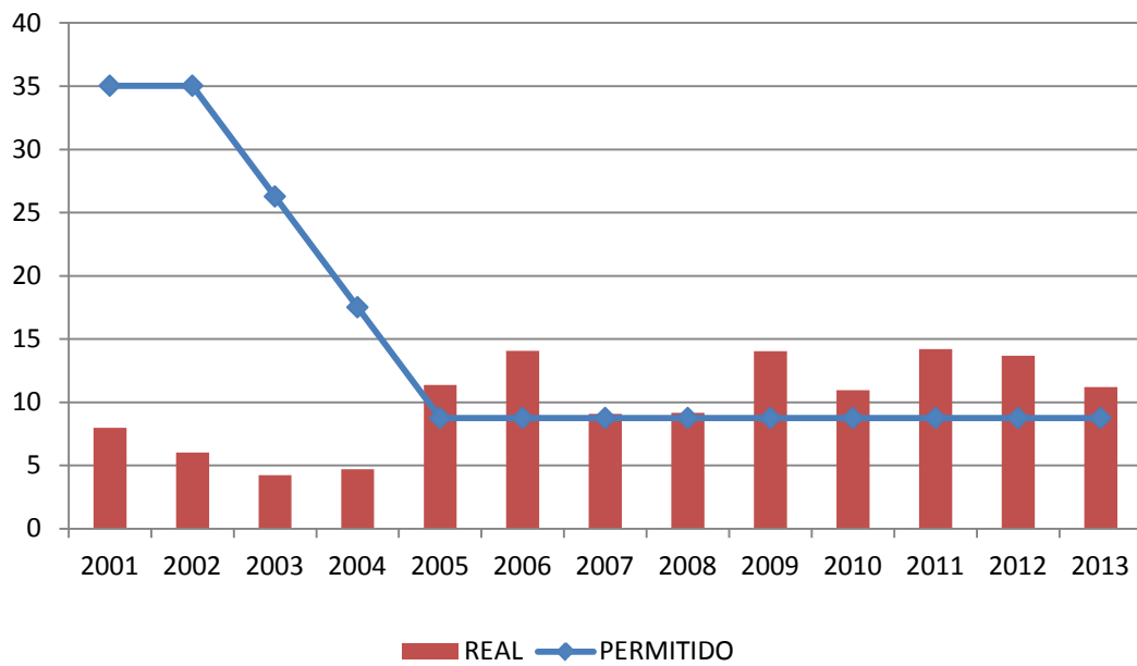
GRÁFICO No. 51 SAIDI DE EDECHI EN CENTROS URBANOS AÑOS 2001 - 2013
