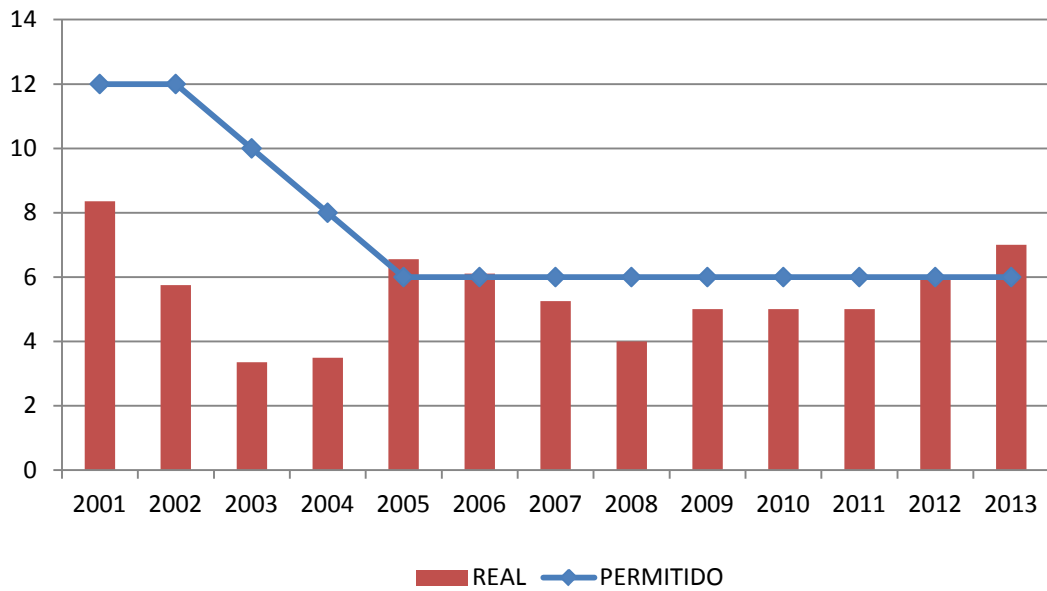
GRÁFICO No. 47 SAIFI DE EDEMET EN CENTROS URBANOS AÑOS 2001 - 2013
