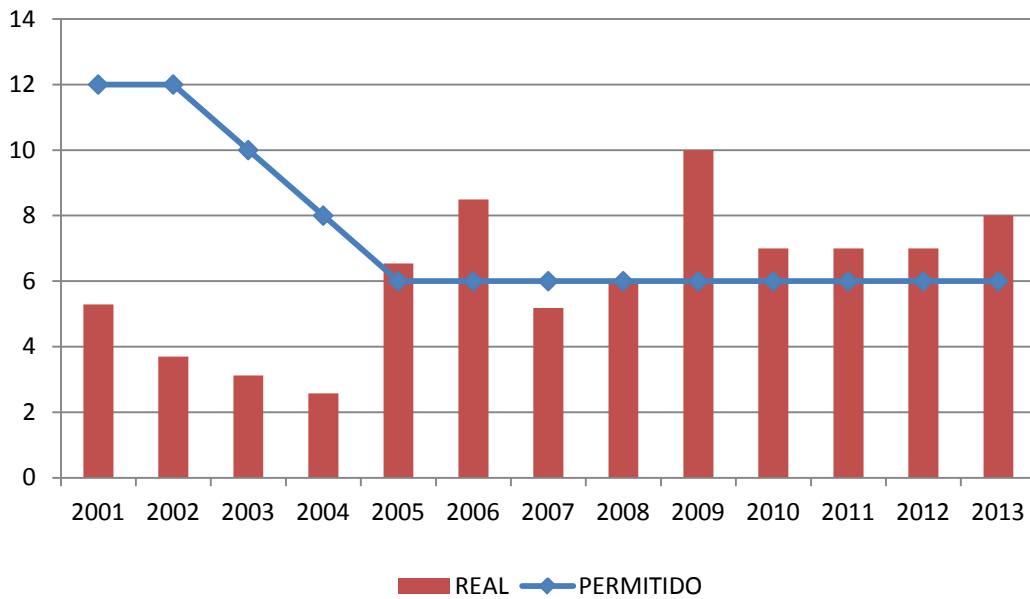
GRÁFICO No. 48 SAIFI DE EDECHI EN CENTROS URBANOS AÑOS 2001 - 2013
