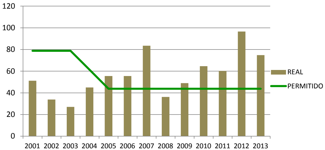
GRÁFICO No. 55 SAIDI DE ENSA EN CENTROS RURALES AÑOS 2001 - 2013
