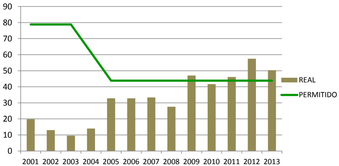
GRÁFICO No. 56 SAIDI DE EDEMET EN CENTROS RURALES AÑOS 2001 - 2013
