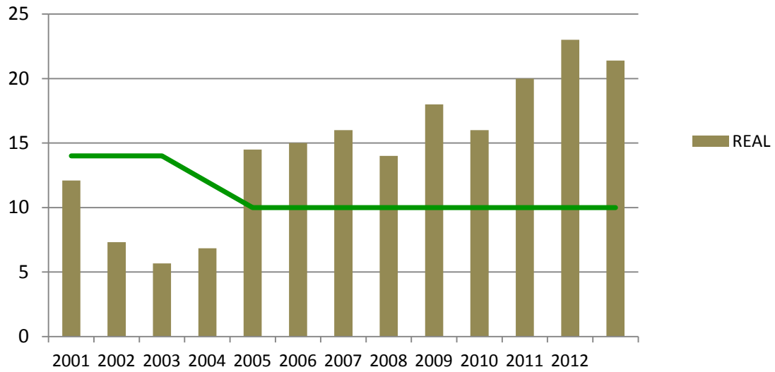
GRÁFICO No. 53 SAIFI DE EDEMET EN CENTROS RURALES AÑOS 2001 - 2013
