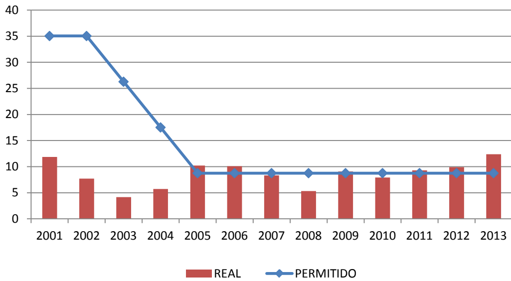
GRÁFICO No. 50 SAIDI DE EDEMET EN CENTROS URBANOS AÑOS 2001 - 2013
