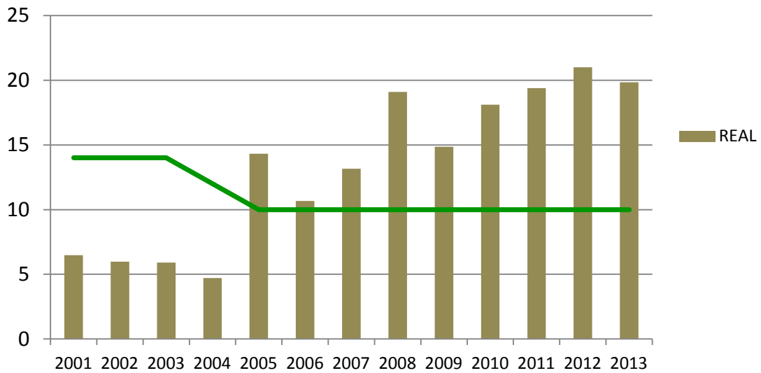
GRÁFICO No. 54 SAIFI DE EDECHI EN CENTROS RURALES AÑOS 2001 - 2013
