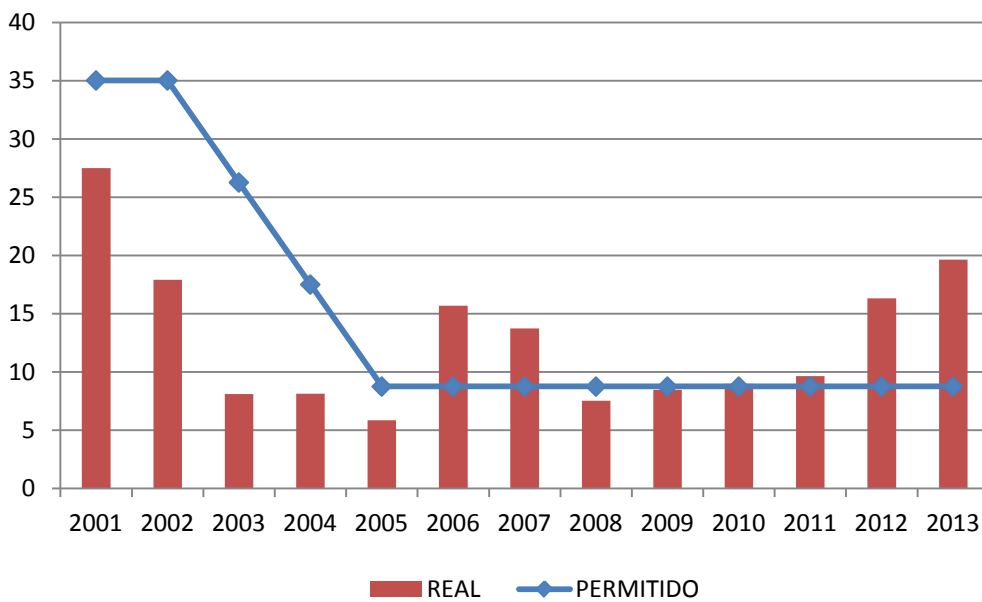
GRÁFICO No. 49 SAIDI DE ENSA EN CENTROS URBANOS AÑOS 2001 - 2013
