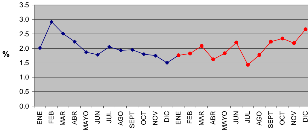
GRÁFICO No. 12 PÉRDIDAS EN EL SISTEMA DE TRANSMISIÓN AÑOS 2006 Y 2007
